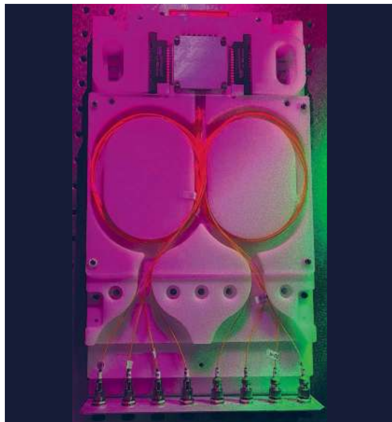
SORGENTE DI STATI ENTANGLED PLUG&PLAY PER DEVICE INDEPENDENT QUANTUM CRYPTOGRAPHY, SVILUPPATO NEI QUANTUM OPTICS LAB DEL DIPARTIMENTO SBAI – SAPIENZA, NELL'AMBITO DEL PROGETTO “QUASAR”.
